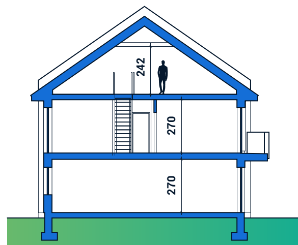
PRZEKRÓJ
