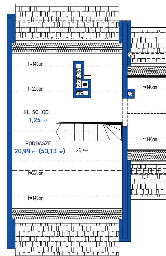
PODDASZE
