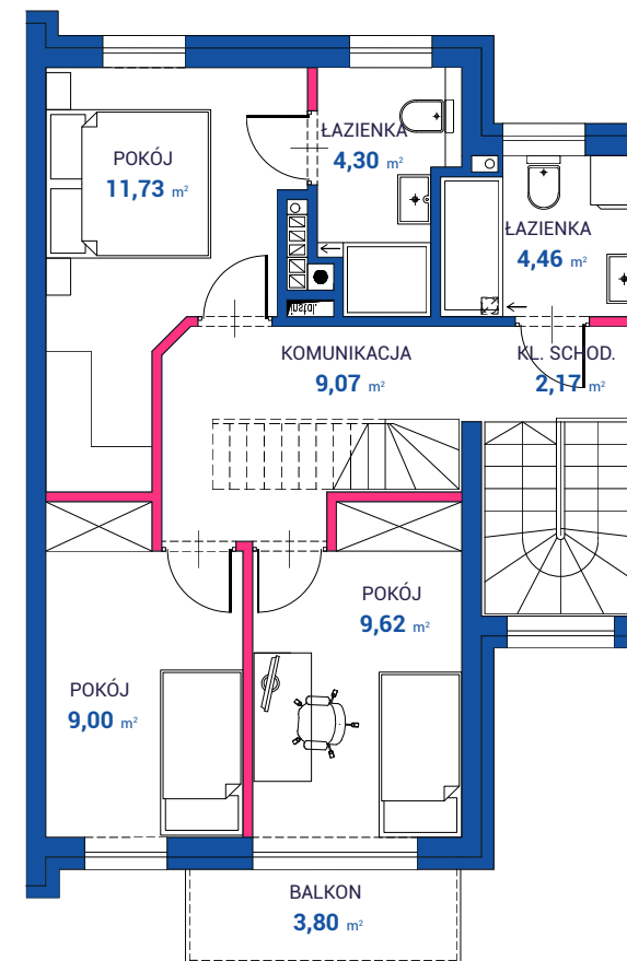
PODDASZE
